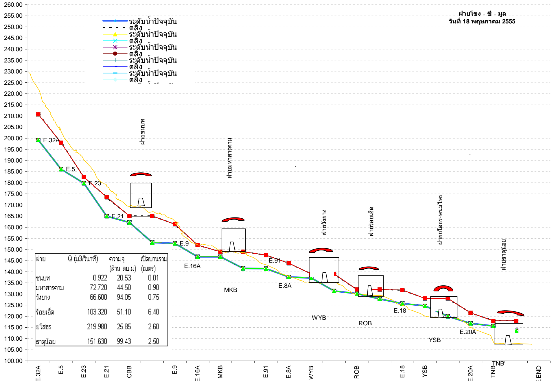
รูปตัดตามยาวแม่น้ำชี และ ระดับน้ำปัจจุบัน
